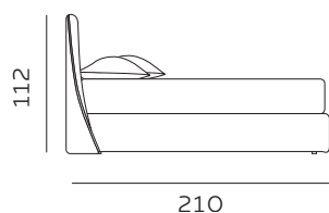
210 materasso lungh. cm. 190 mattress length cm. 190
