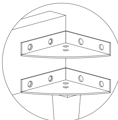
Dettaglio A, Scala 1:5 / Detail A, Scale 1:5
