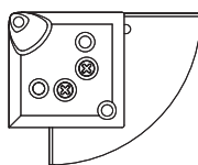
Piedino posteriore destro Vedi dettaglio C Right rear foot See detail C
