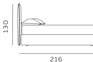
216 materasso lungh. cm. 200 mattress length cm. 200
