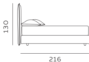
materasso lungh. cm. 200 mattress length cm. 200
