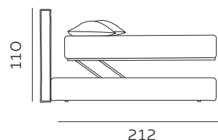
212 materasso lungh. cm. 190 mattress length cm. 190
