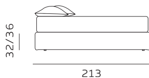
materasso lungh. cm. 200 mattress length cm. 200
