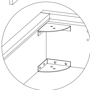
Dettaglio A Scala 1:10 Detail A Scale 1:10
