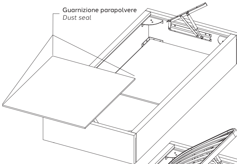
Dettaglio D Scala 1:10 Detail D Scale 1:10
