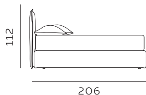
206 materasso lungh. cm. 190 mattress length cm. 190
