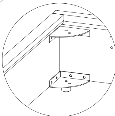
Dettaglio B Scala 1:10 Detail B Scale 1:10
